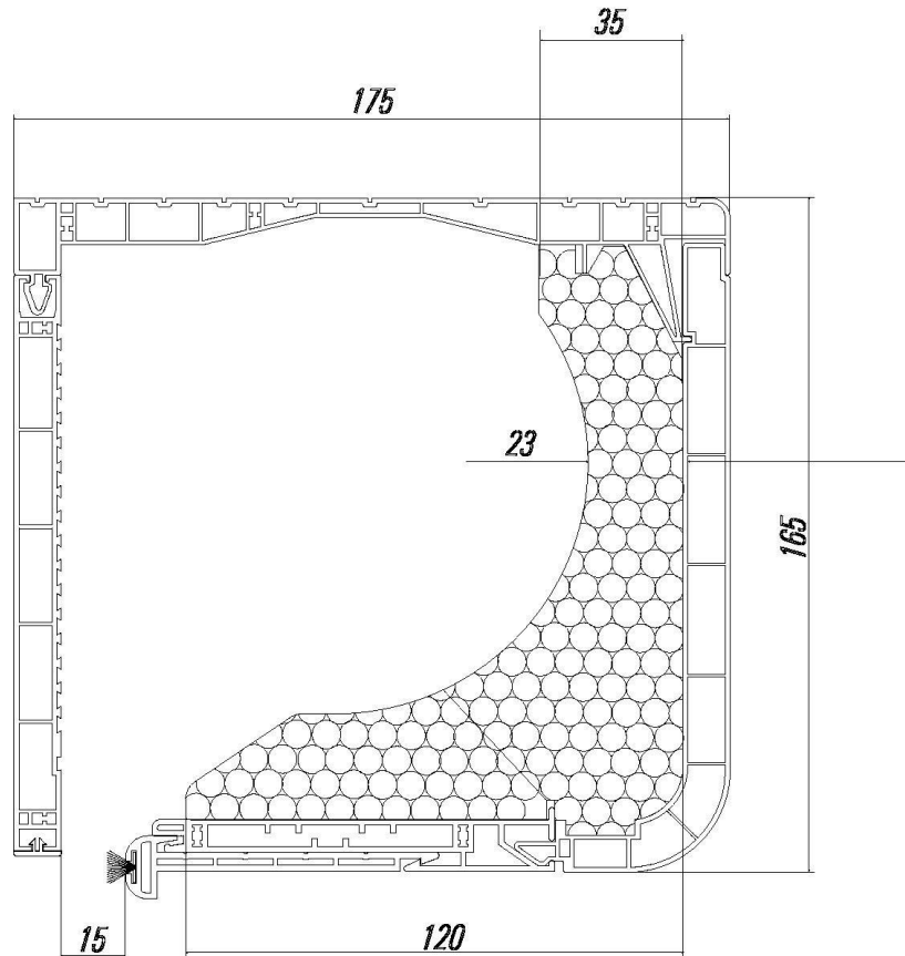
Bild 2 Schnittzeichnung
